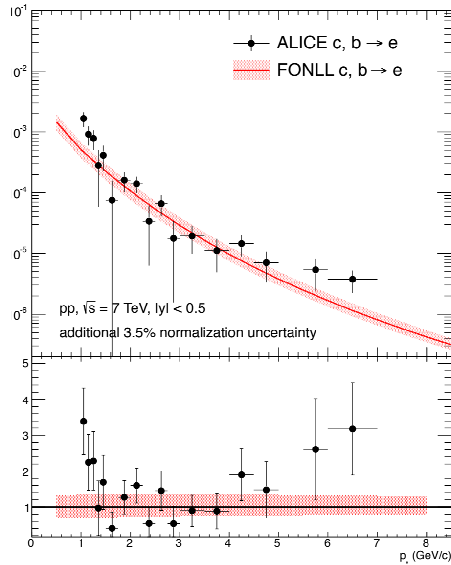
TPC+TOF (sec 2,3,4,5)
